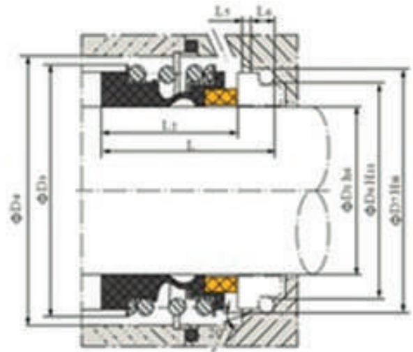
Schéma PIM2
