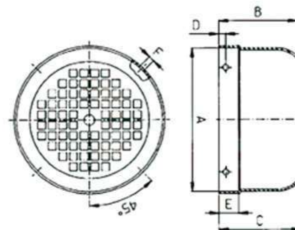
schéma CVP
