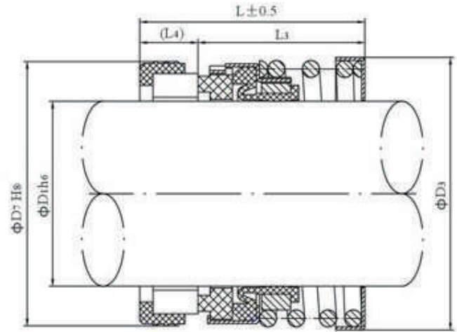
Schéma P960
