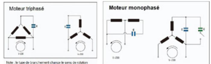
Condensateur pour moteur avec double cosses
