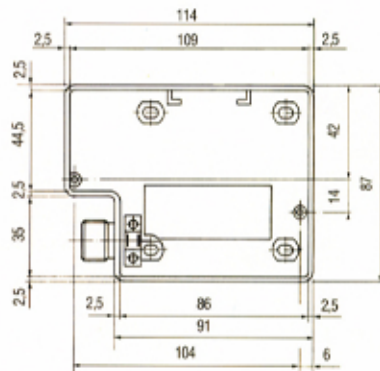
Sez. A-A
